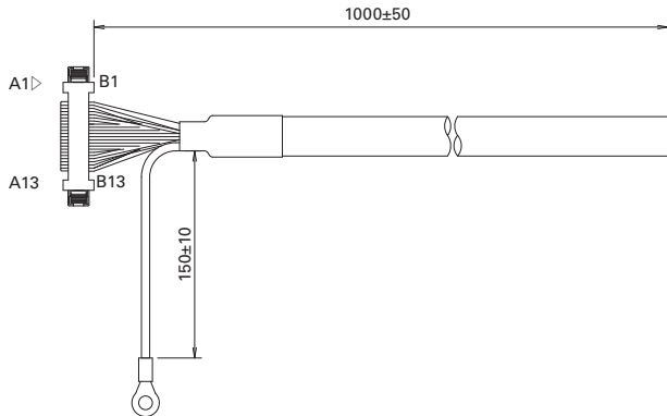
CN wiring
